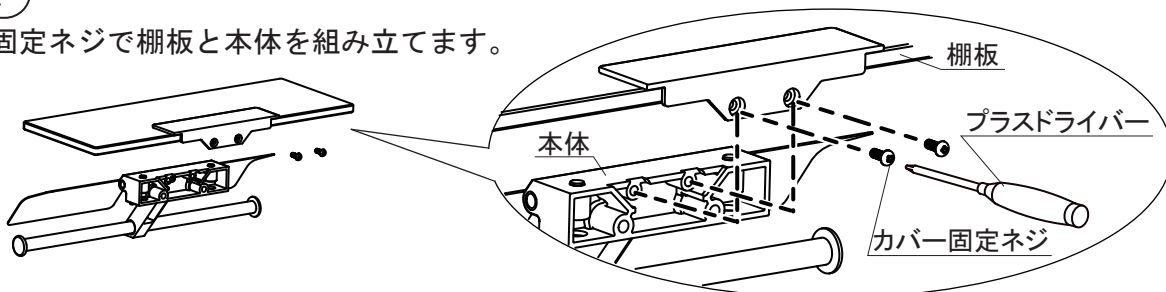
カバー固定ネジ 2本 (ナベ小ネジ M4×10)
