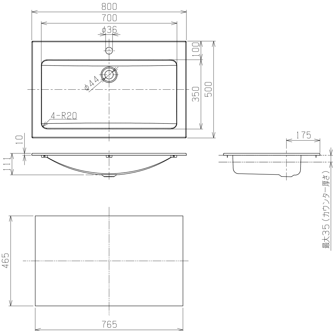
カウンター切込寸法図
