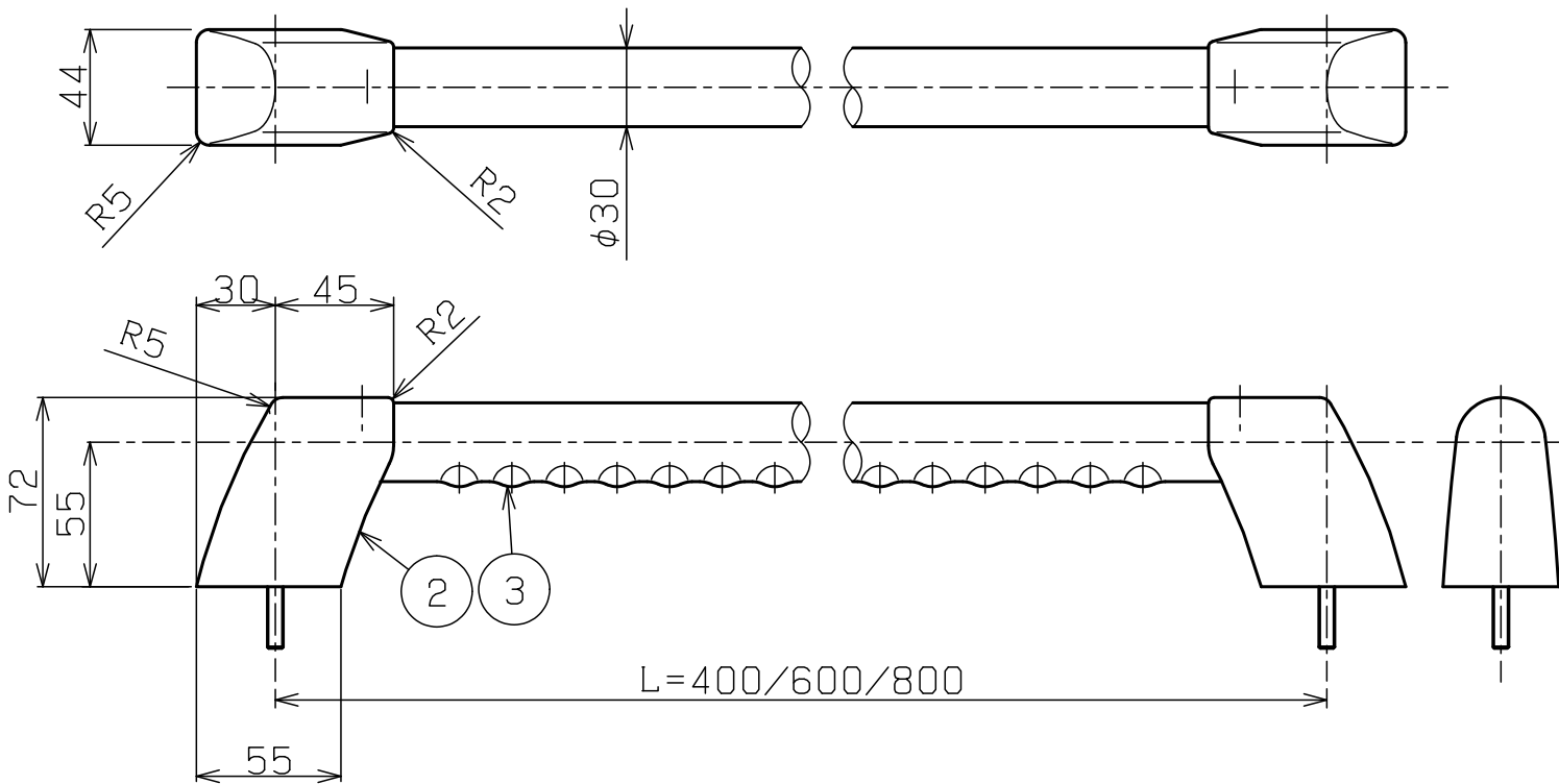
Aタイプ・Bタイプ取付ネジピッチ
