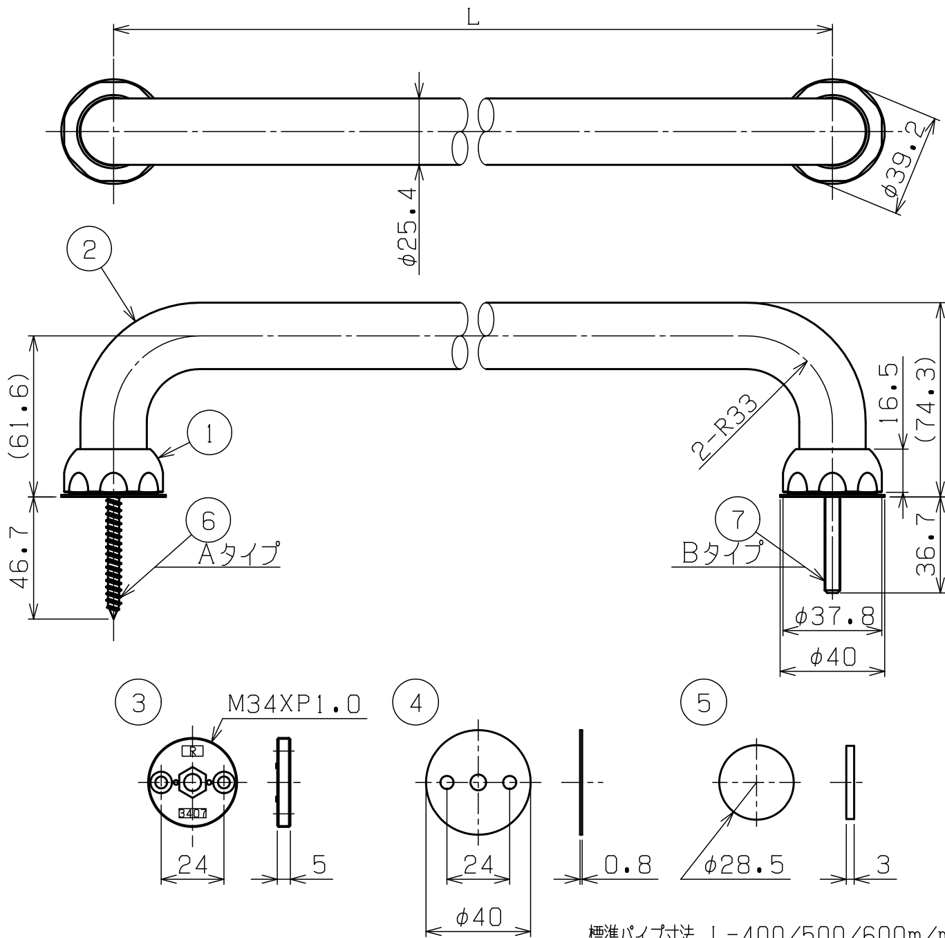
標準パイプ寸法 L-400/500/600m/m
